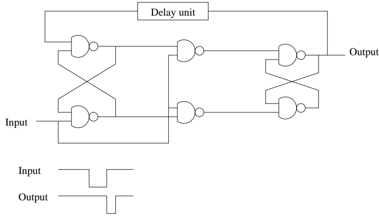
Figure 6: Edge detector.
